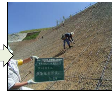
鉄筋組立
